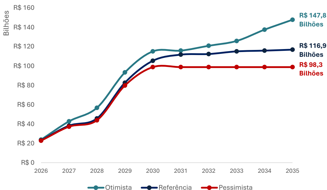
Figura 4-19 – Cenários de expansão do sistema de transmissão
